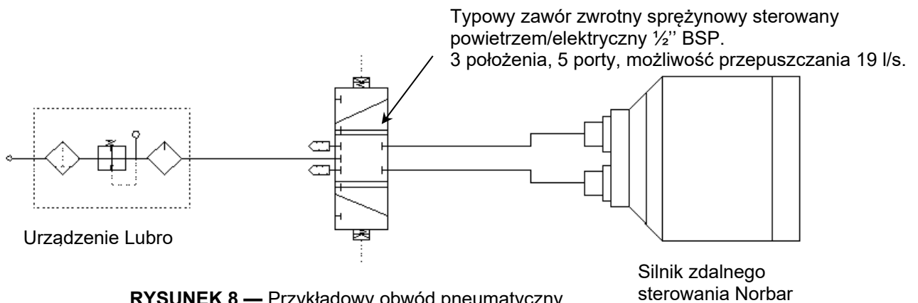
RYSUNEK 8 — Przykładowy obwód pneumatyczny
