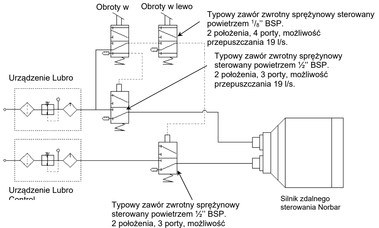
RYSUNEK 7 — Przykładowy obwód pneumatyczny
