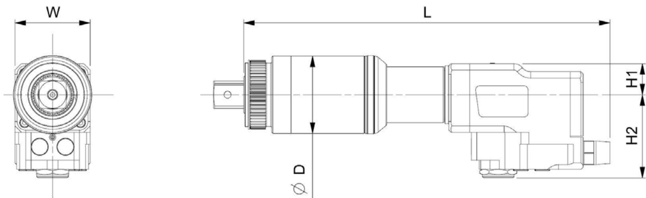
AFBEELDING 13 – afmetingen
