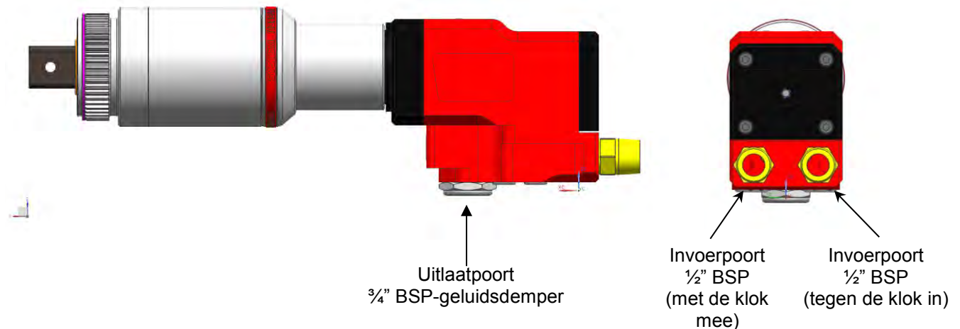
AFBEELDING 9 – poorten
