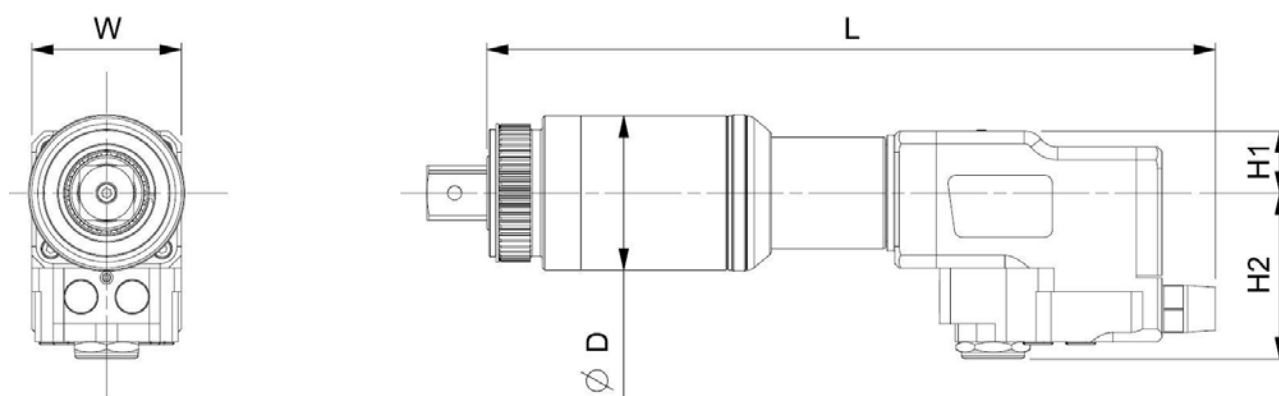
FIGUR 13 – Dimensioner
