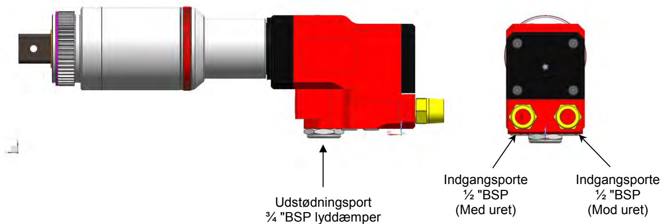
FIGUR 9 - Porte
