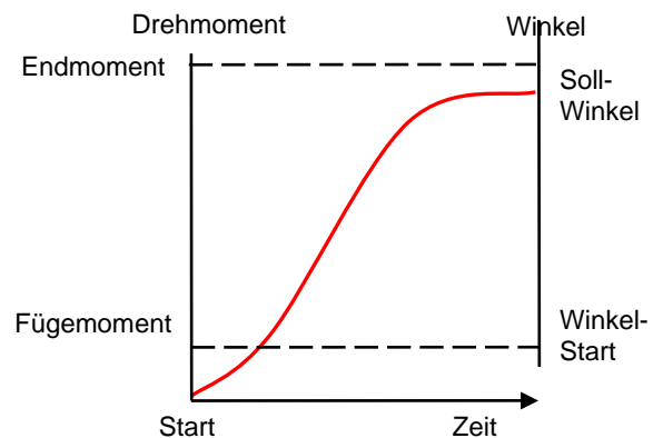
ABBILDUNG 50 – Winkelmodus
