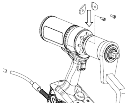
ABBILDUNG 4 – Einlegeplatten montieren
