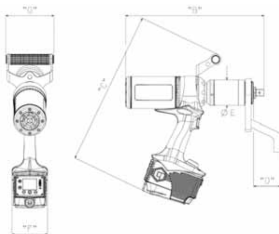
ABBILDUNG 57 – Werkzeugabmessungen
